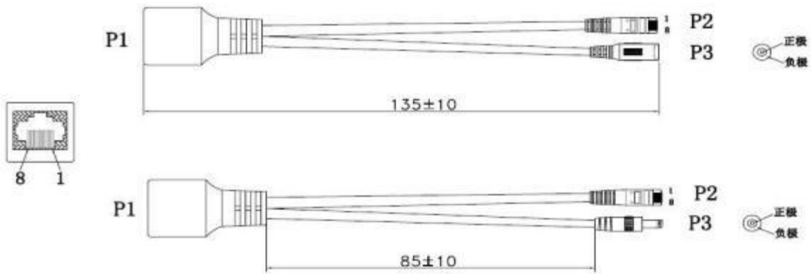
接线图
